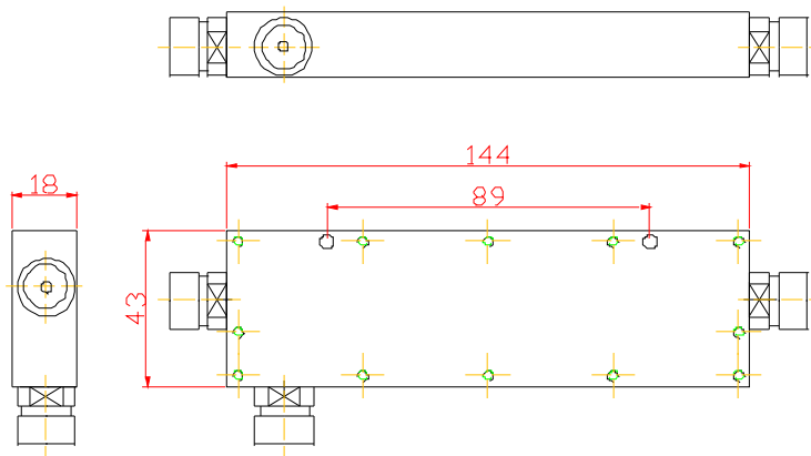
Outline Drawing(Unit:mm)
