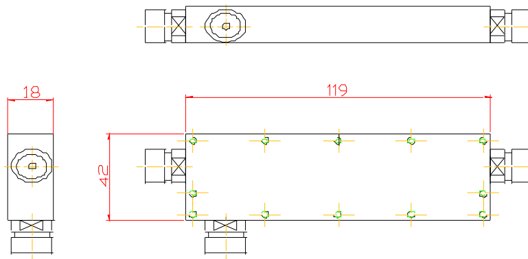
Outline Drawing(Unit:mm)
