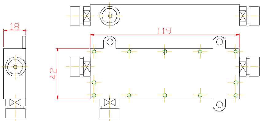
Outline Drawing(Unit:mm)
