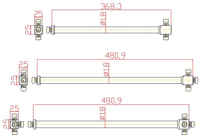
Outline Drawing(Unit:mm)
