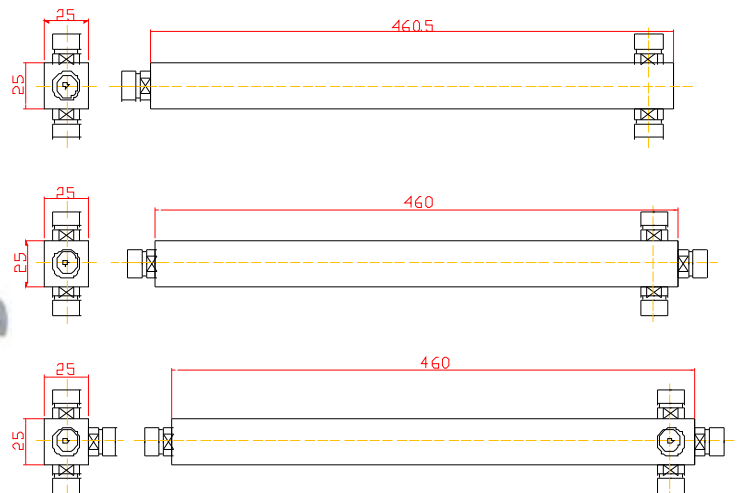
Outline Drawing(Unit:mm)
