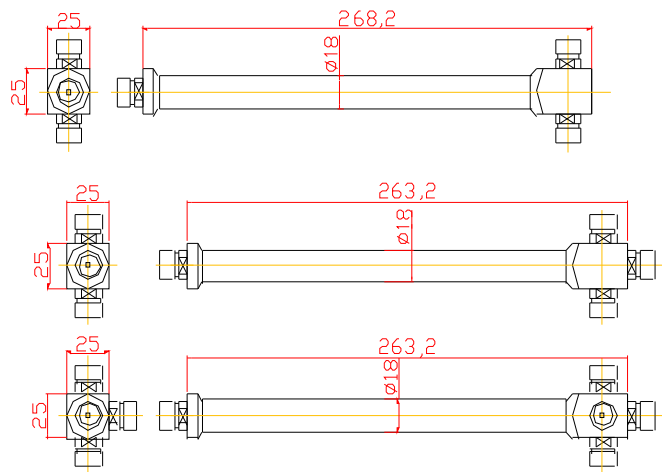
Outline Drawing(Unit:mm)
