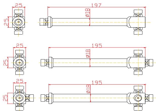
Outline Drawing(Unit:mm)
