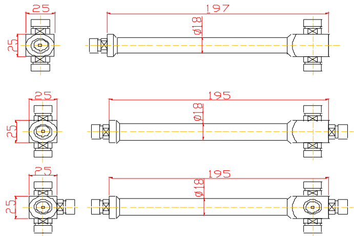
Outline Drawing(Unit:mm)
