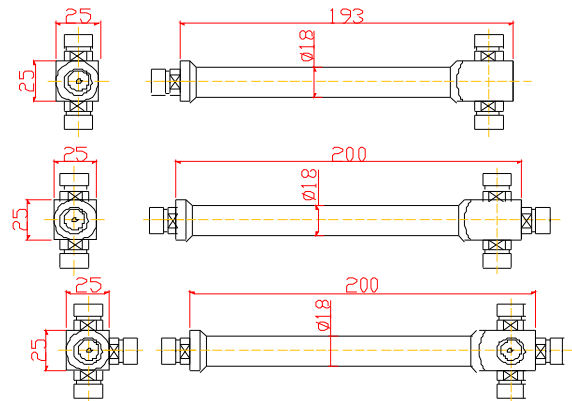
Outline Drawing(Unit:mm)
