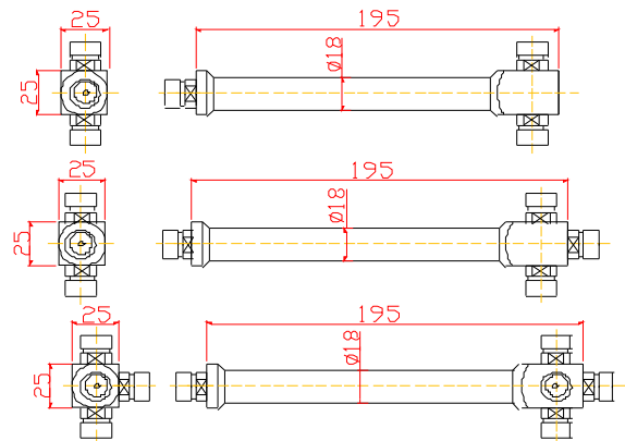
Outline Drawing(Unit:mm)
